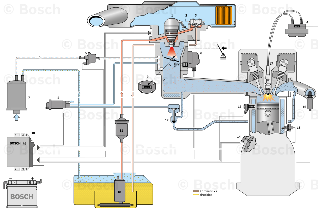
Systembild einer Mono-Motronic
