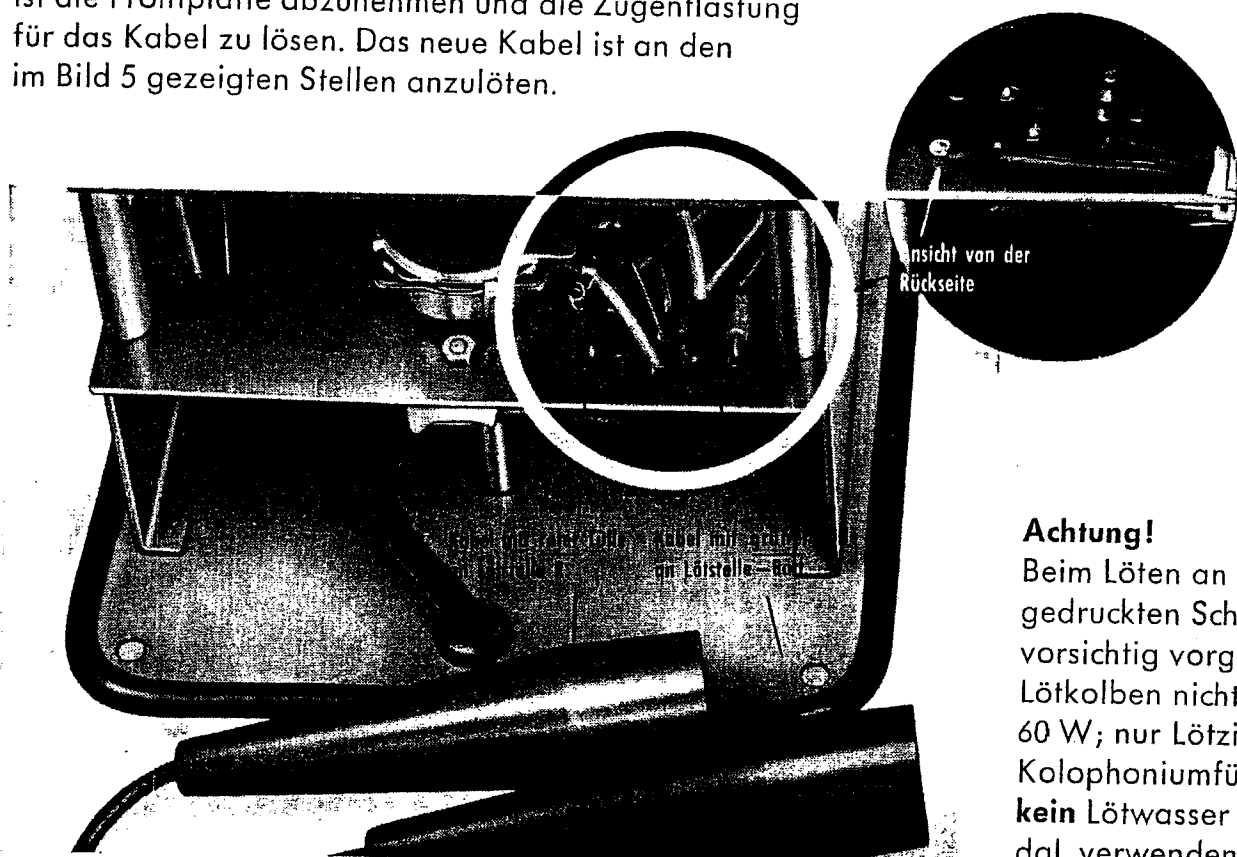
Bild 5 Lötanschlüsse des Testkabels
