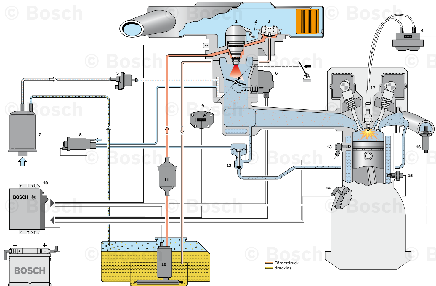
Systembild einer Mono-Motronic
